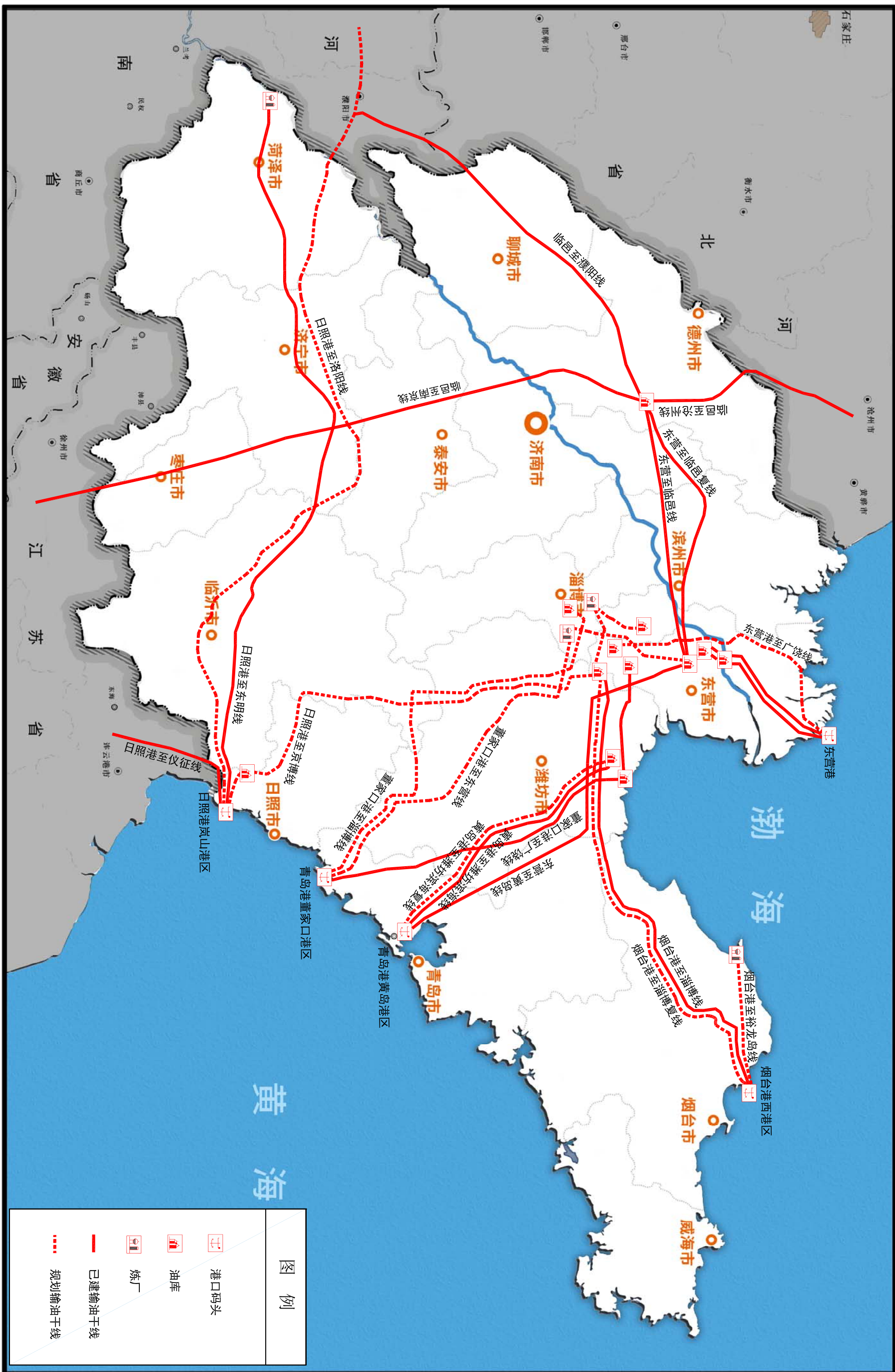
附图4 山东省“十四五”原油管网布局示意图
